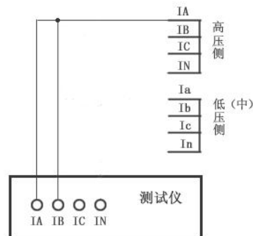
三相电流接线
