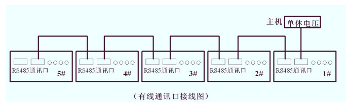
图 2.4.4.4 有线通讯接口接口图
