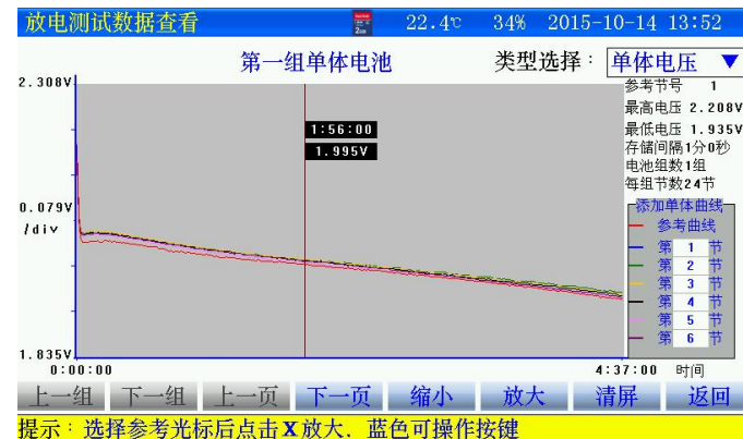
图 3.7.4-1 单体电压曲线界面
